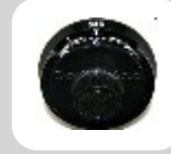
Serrure à disques S&G 8550 Groupe 1 silencieuse intôtatable 800 000 combinaisons Argos classe C SGN
